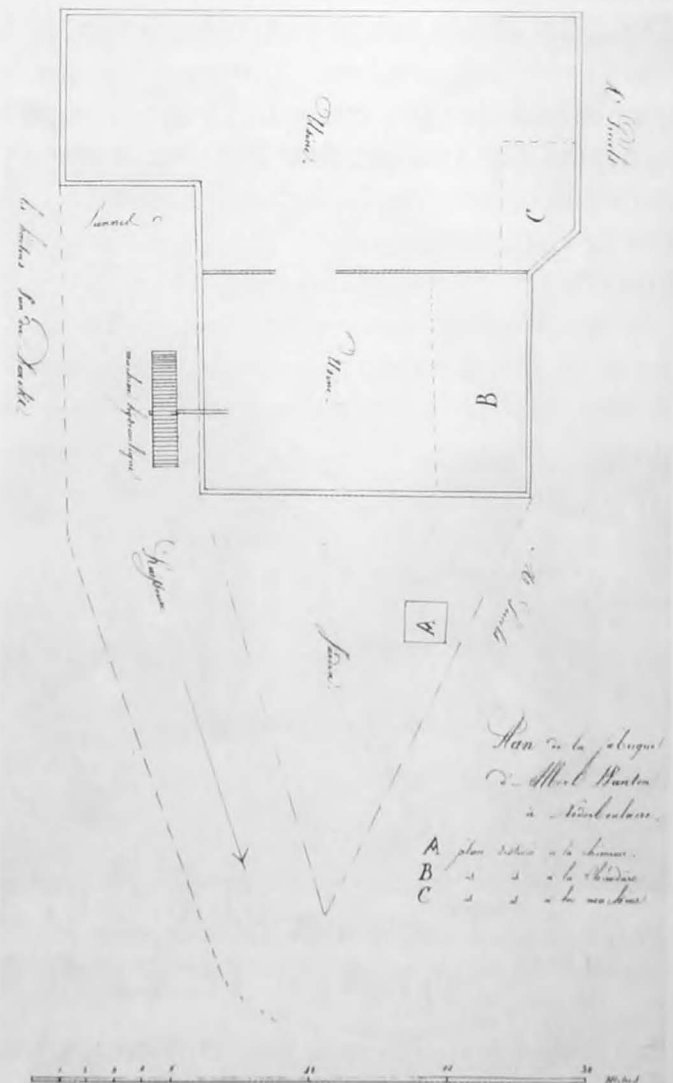
Afb. 13: grondplan van de katoenweverij van A. Wanten met plaatsaanduiding van stoommachine, -ketel en fabrieksschouw (1838)
