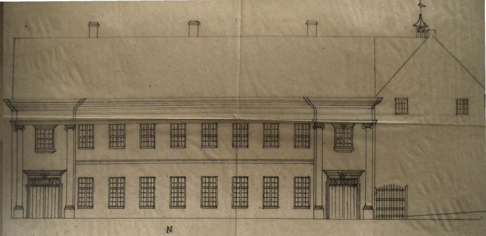
Ontwerp van de voorgevel van de lucifersfabriek van 'Egidius Coppens en Cie' in de Gentsestraat te Nederboelare (12 juli 1858).
